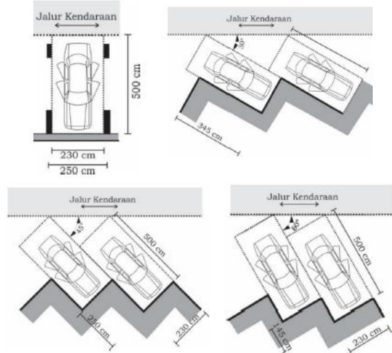
Gambar 4.24 Dimensi bentuk ruang parkir
