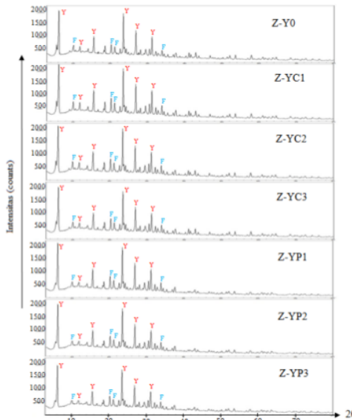
Gambar 2. Difraktogram XRD zeolit hasil sintesis dengan waktu hidrotermal 72 jam
