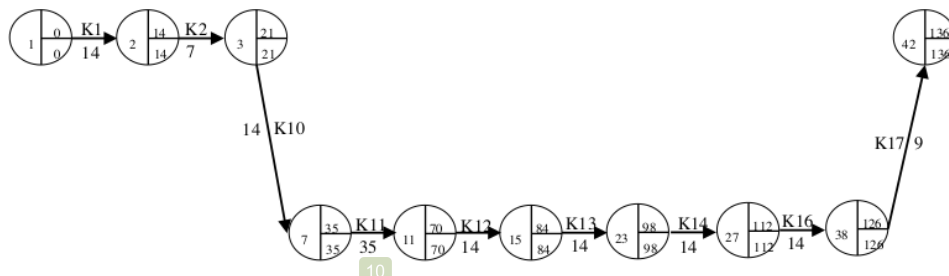
Gambar 1. NWP lintasan kegiatan K1, K2, K10, K11, K12, K13, K14, K16 dan K17 (lintasan kritis).
