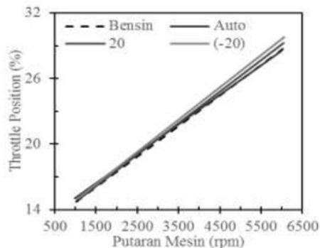
Gambar 3. Grafik hubungan throttle position terhadap putaran mesin
