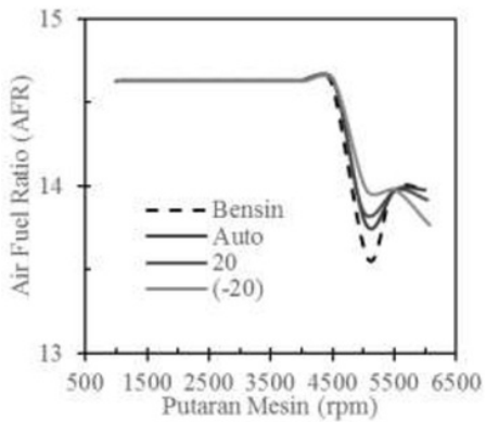
Gambar 7. Grafik hubungan AFR terhadap putaran mesin
