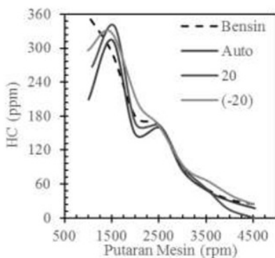
Gambar 8. Grafik hubungan emisi HC terhadap putaran mesin
