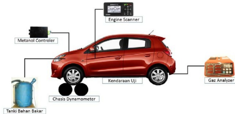
Gambar 2. Skema peralatan pengujian
