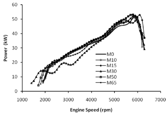
Gambar 6. Perbandingan daya untuk berbagai komposisi metanol
