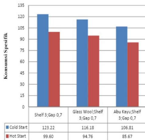
Gambar 3.4. Hubungan konsumsi spesifik terhadap jenis isolator
