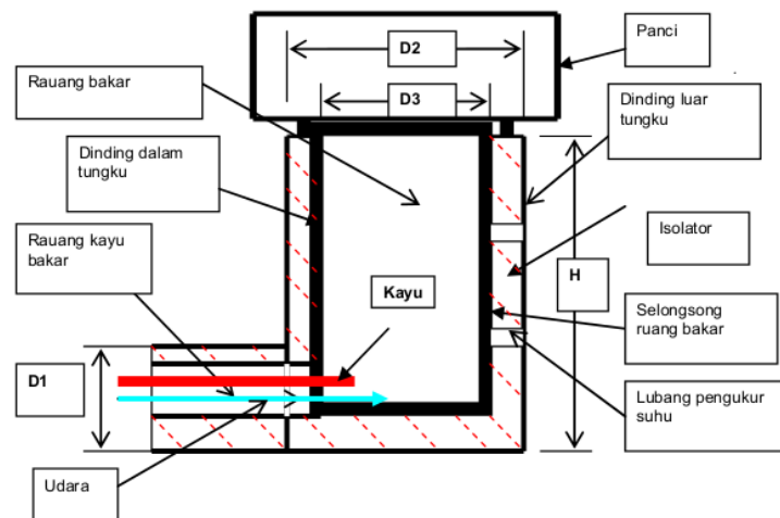
Gambar 2. 1. Tungku bahan bakar kayu
