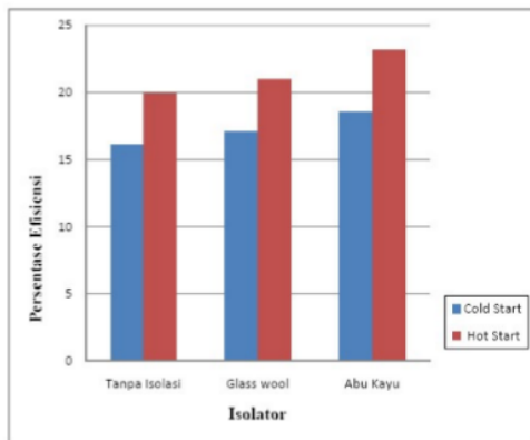
Gambar 3.3. Hubungan efisiensi terhadap jenis isolator
