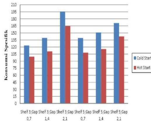
Gambar 3.2. Hubungan konsumsi spesifik terhadap posisi tinggi rak (shelf) dan jarak panci (gap) pada tungku tanpa isolator.
