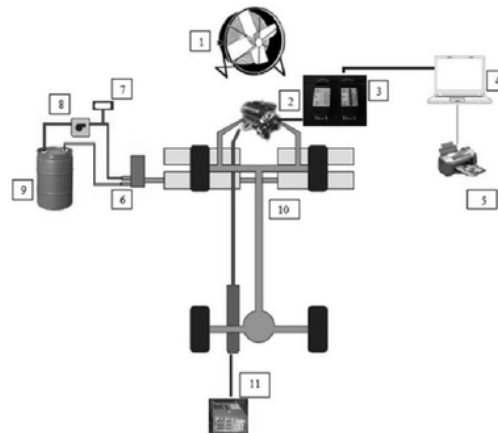
Gambar 1. Susunan Alat Uji di Laboratorium
