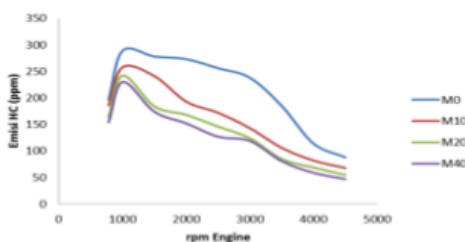
Gambar 6 : Pengaruh Penambahan Metanol Terhadap Emisi HC.
