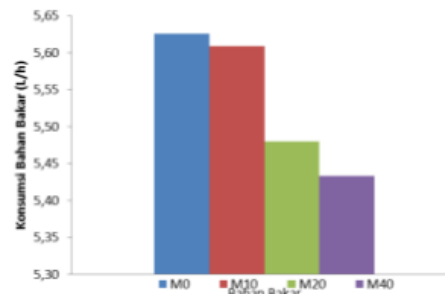
Gambar 4. Rata-rata Konsumsi Bahan Bakar
