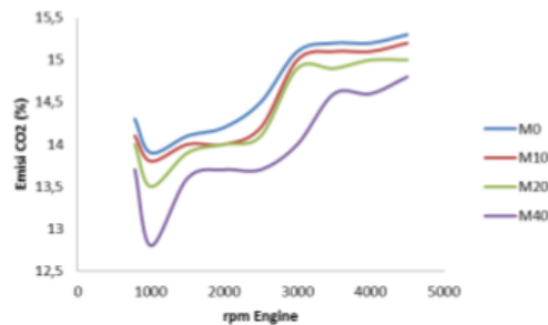
Gambar 8 : Pengaruh Penambahan Metanol Terhadap Emisi CO 2 .
