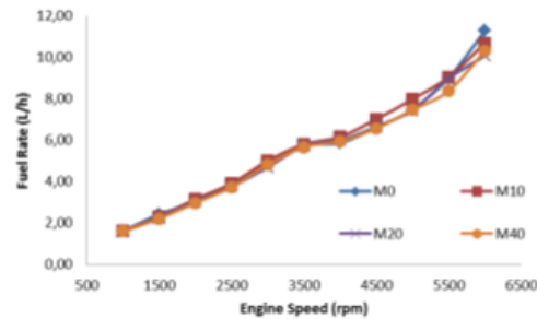
Gambar 3 : Pengaruh Penambahan Metanol Terhadap Konsumsi Bahan Bakar
