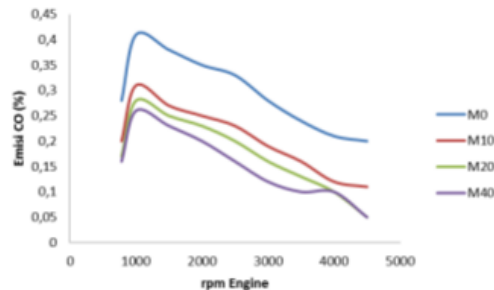
Gambar 7 : Pengaruh Penambahan Metanol Terhadap Emisi CO.
