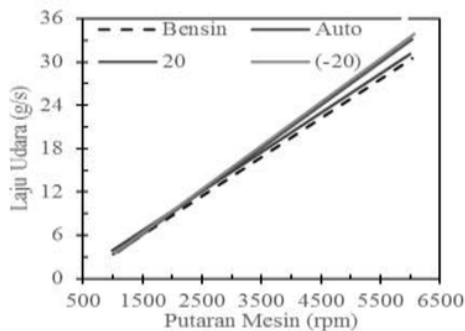
Gambar 4. Grafik hubungan laju udara terhadap putaran mesin
