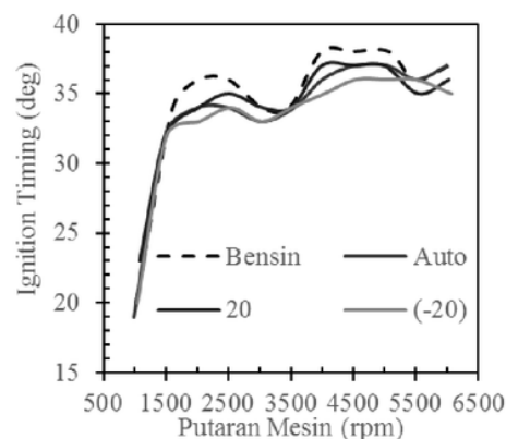
Gambar 6. Grafik hubungan ignition timing terhadap putaran mesin
