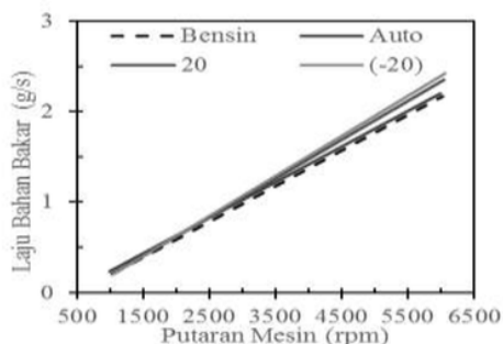
Gambar 5. Grafik hubungan laju bahan bakar terhadap putaran mesin
