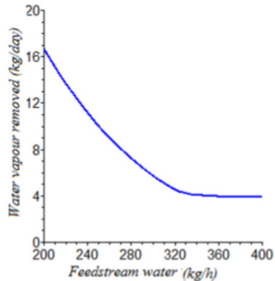
Gambar 5. Grafik Pengaruh water feedstream terhadap kerja cooler
