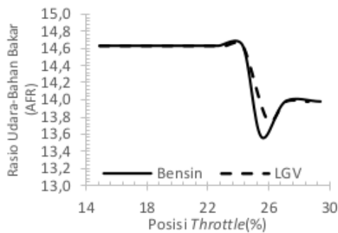
Gambar 9. Grafik hubungan rasio udara-bahan bakar terhadap posisi throttle di mobil Mitsubishi Mirage.
