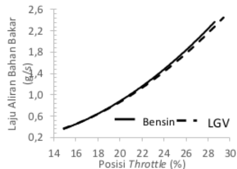
Gambar 11. Grafik hubungan laju aliran bahan bakar terhadap posisi throttle di mobil Mitsubishi Mirage.
