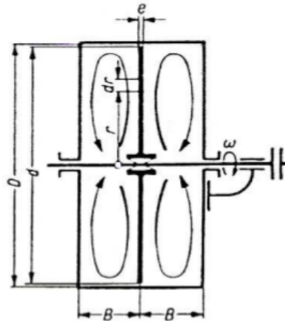
Gambar 2. Perputaran Air Pada Disk
