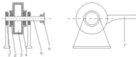
Gambar 1. Konstruksi Dynamometer Hidrolik
