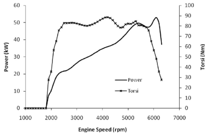
Gambar 4. Kurva torsi dan daya dengan bahan bakar M15
