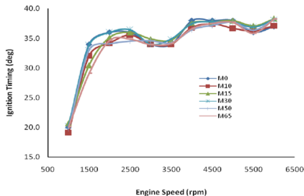
Gambar 10. Waktu penyalaan untuk berbagai campuran metanol
