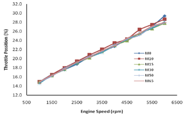
Gambar 7. Posisi throttle saluran udara untuk berbagai campuran metanol
