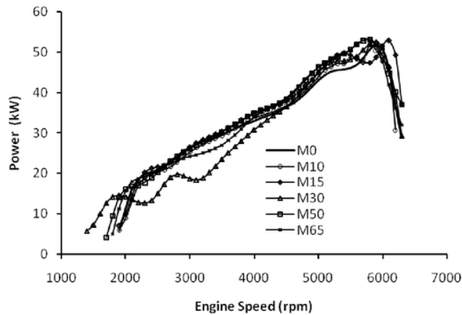
Gambar 6. Perbandingan daya untuk berbagai komposisi metanol
