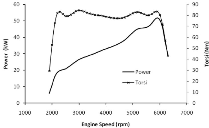
Gambar 3. Kurva torsi dan daya dengan bahan bakar bensin murni
