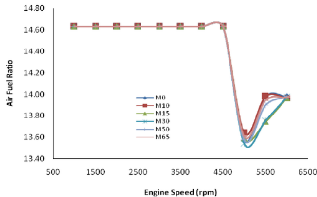
Gambar 9. Rasio udara-bahan bakar untuk berbagai campuran metanol
