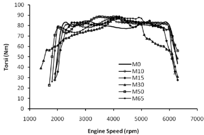
Gambar 5. Perbandingan torsi untuk berbagai komposisi metanol
