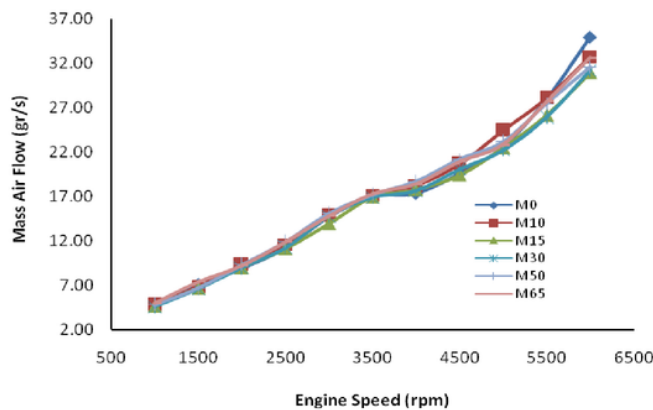
Gambar 8. Laju aliran massa udara untuk berbagai campuran metanol
