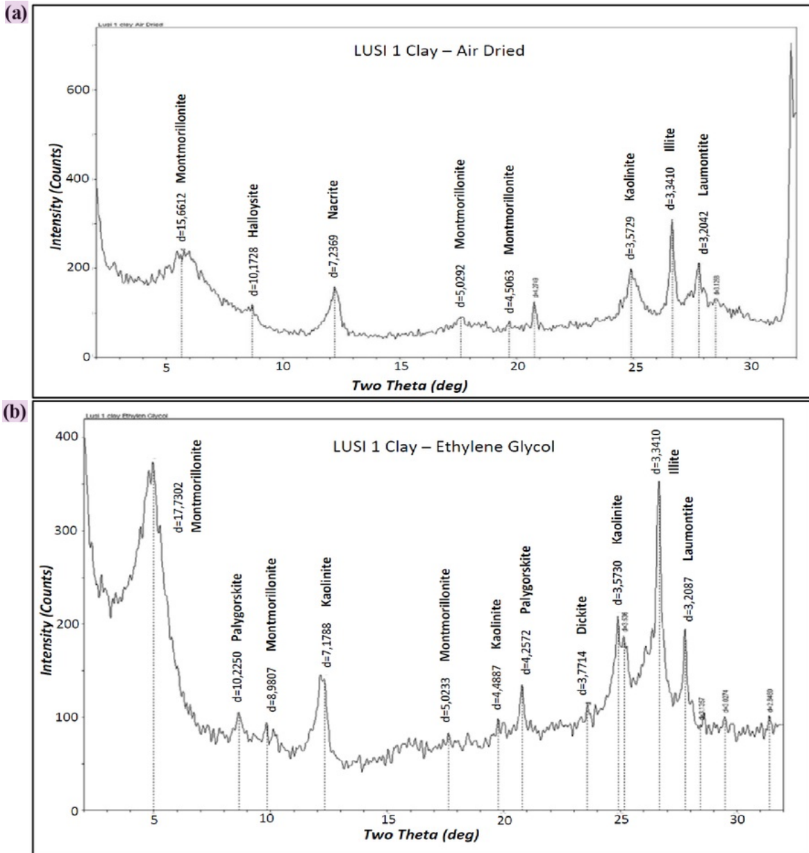
Gambar 3. Contoh grafik hasil analisis XRD menunjukkan puncak kemunculan mineral lempung tertentu, perbandingan perlakuan air dried (a) dan etilen glikol (b) pada sampel Lusi 1.
