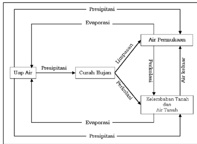
Gambar 1. Siklus Hidrologi dalam Metode Mock Sumber: Mock (1973)
