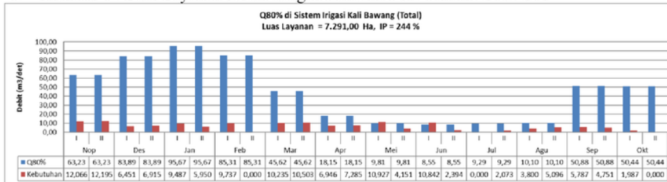
Gambar 4. Neraca Air di Sistem Irigasi Kalibawang (Sesuai Rencanan Pola Tanam 2015/2016)
