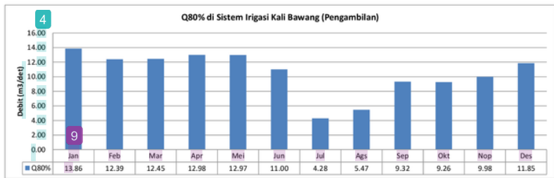
Gambar 3. Debit Andalan Total di Sistem Irigasi Kalibawang
