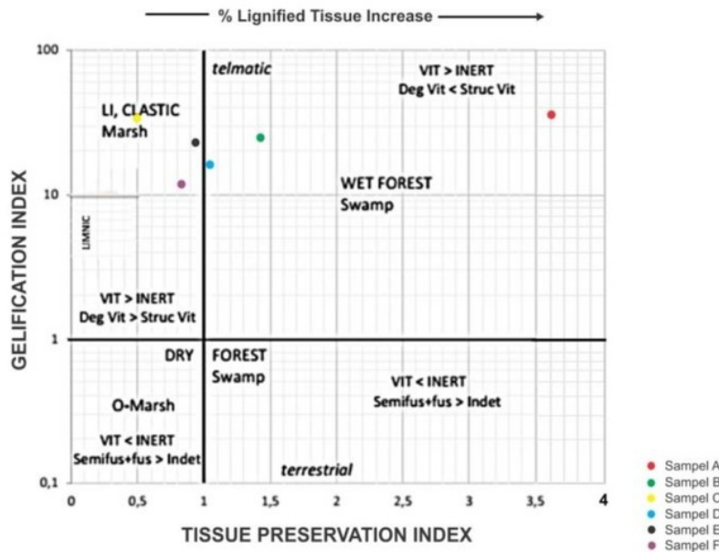
Gambar 9. Hasil plotting pada diagram TPI-GI (dimodifikasi dari Diessel, 1986, dalam Lamberson, 1991).
