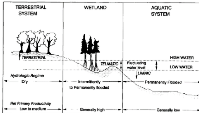
Gambar 3. Kondisi lingkungan pengendapan batubara (Mitsch dan Geosselink, 1986 dalam Lamberson dkk., 1991)
