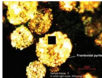
Gambar 7. Fotomikrograf framboidal pyrite pada sampel F.
