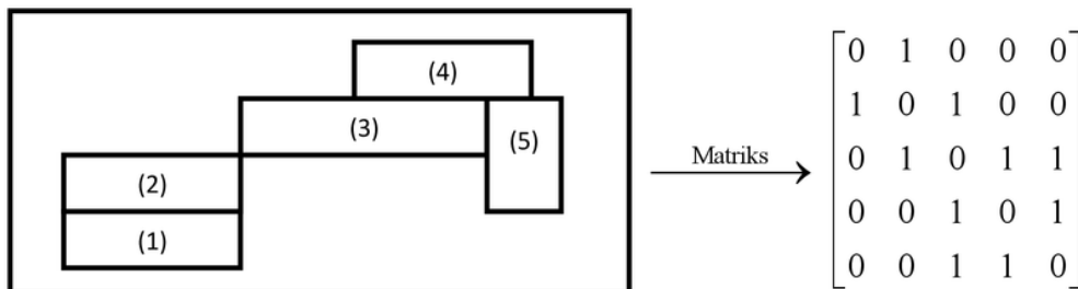
Gambar 1. Ilustrasi Perhitungan Matriks Pembobot Contiguity
