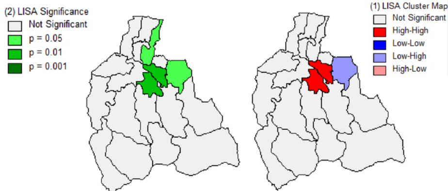
Gambar 6. Peta Signifikansi LISA dan Pengelompokkan Kecamatan April 2010
