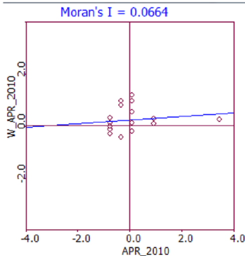
Gambar 5. Moran's Scatterplot penderita DBD pada bulan April 2010
