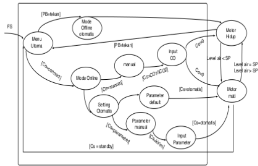
Gambar 6 Diagram state sistem pengendalian ketinggian level cairan.
