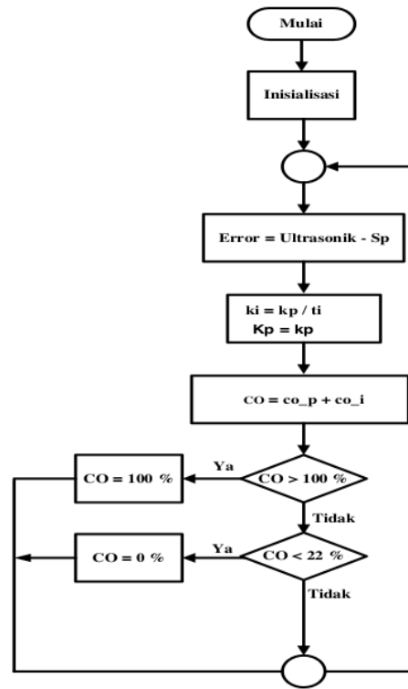
Gambar 7 Diagram alir perhitungan pengendali PI
