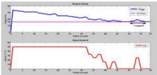
Gambar 17 Respon sistem kontrol PI terhadap gangguan.
