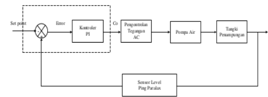
Gambar 5 Diagram blok sistem pengendalian level ketinggian cairan
