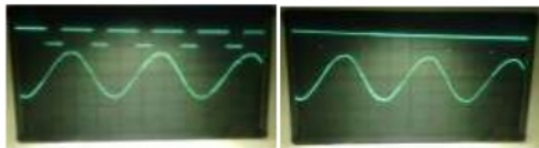
Gambar 9 Bentuk gelombang untuk sinyal kontrol 60% dan 100%.
