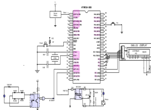
Gambar 3 Alokasi port pada sistem minimum mikrokontroler Atmega 8535.
