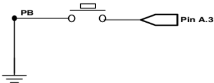
Gambar 4 Alokasi port untuk push button.
