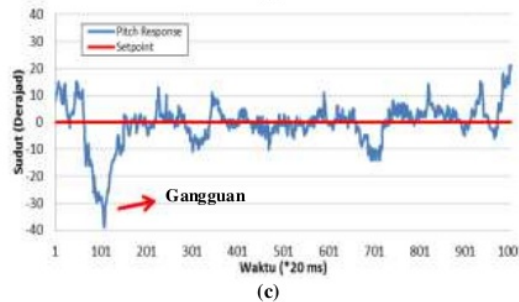
Gambar 13. Respon sistem dengan gangguan ke bawah : (a) Respon sistem dengan variasi ke-1 ( \pm 12^0 ) (b) Respon sistem dengan variasi ke-2 ( \pm 10^0 ) (c) Respon sistem dengan variasi ke-3 ( \pm 8^0 )
