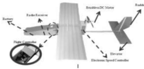
Gambar 3. Desain mekanik untuk pengujian terbang.
