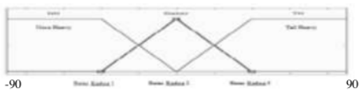
Gambar 7. Himpunan keanggotaan masukan sudut pitch complementary filter ( \theta )
