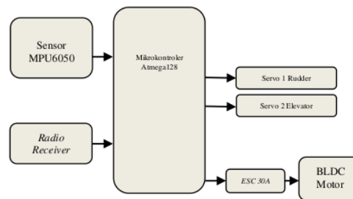
Gambar 1 Desain sistem elektronika pada UAV
