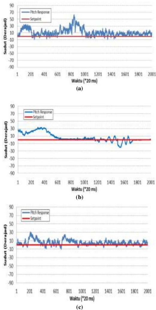
Gambar 14. Respon kontrol sistem secara keseluruhan: (a) Respon sistem dengan variasi ke-1 ( \pm 12^\circ ) (b) Respon sistem dengan variasi ke-2 ( \pm 10^\circ ) (c) Respon sistem dengan variasi ke-3 ( \pm 8^\circ )
