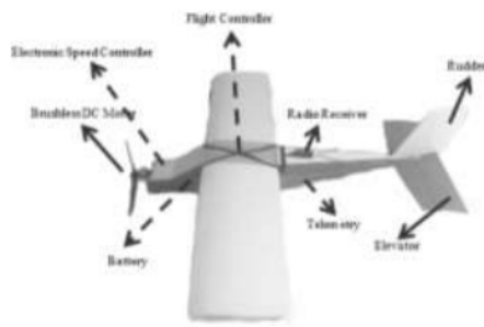
Gambar 2. Desain mekanik untuk pengujian metode kontrol fuzzy
