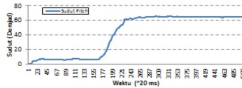
Gambar 11. Grafik respon kontrol open loop sistem UAV
