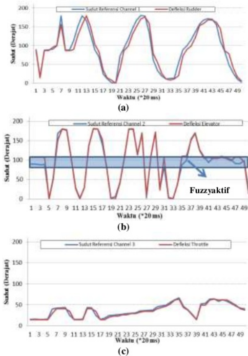
Gambar 8. Grafik respon sinyal masukan aktuator dan sinyal referensi dari radio receiver (a) Grafik perbandingan masukan dari Channel 1 dan keluaran rudder. (b) Grafik perbandingan masukan dari Channel 2 dan keluaran elevator. (c) Grafik perbandingan masukan dari Channel 3 dan keluaran throttle.
