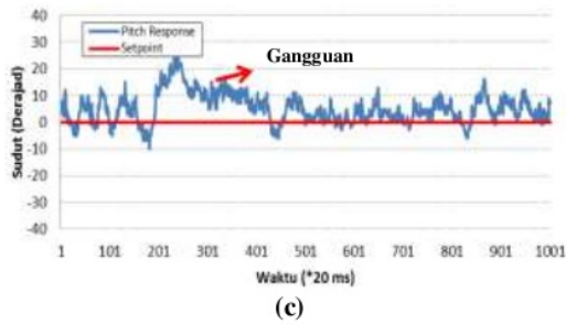
Gambar 12. Respon sistem dengan gangguan ke atas : (a) Respon sistem dengan variasi ke-1 ( \pm 12^0 ) (b) Respon sistem dengan variasi ke-2 ( \pm 10^0 ) (c) Respon sistem dengan variasi ke-3 ( \pm 8^0 )
