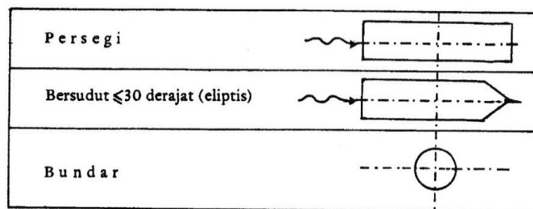
Gambar 2.4 Bentuk/Denah Pilar Dari PPJJR1987
