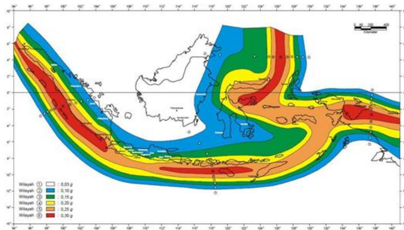
Gambar 2.2 Lokasi Pembagian Daerah Gempa Dari PPJR Tahun 1987
