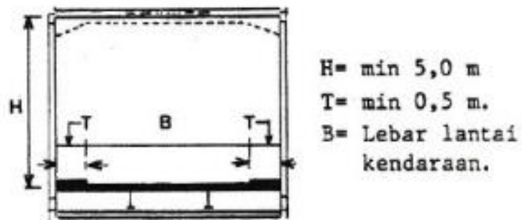
Gambar 2.6 Lebar Maksimum Jembatan Dari PPJJR 1987
