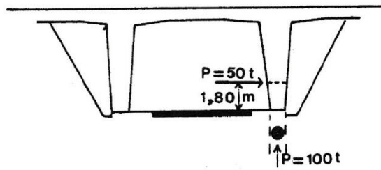
Gambar 2.3 Gaya Tumbuk Pada Jembatan Dari PPIJR 1987
