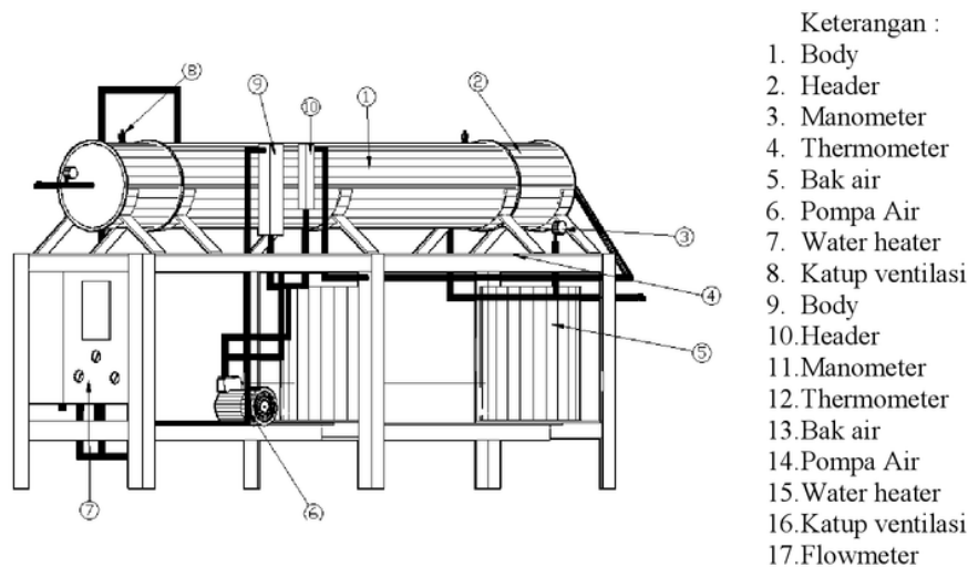
Gambar 2. Gambar Peralatan
