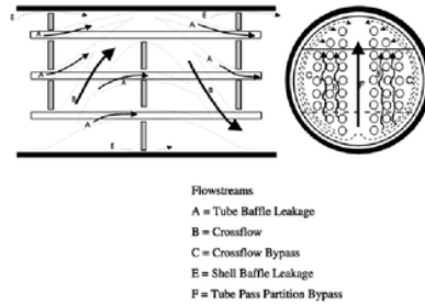
Gambar 3. Aliran fluida ketika melintasi baffle
