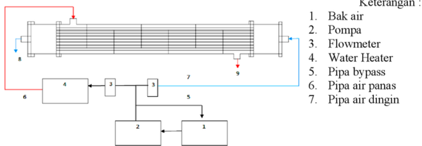
Gambar 1. Skema aliran fluida
