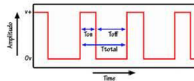
Gambar 2 Contoh Aplikasi PWM
