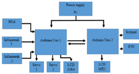
Gambar 5. Blok Diagram Sistem
