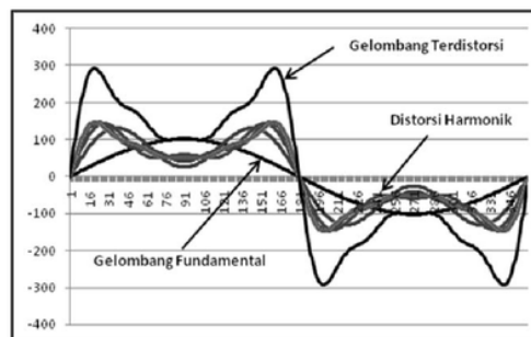
Gambar 1. Gelombang terdistorsi harmonik
