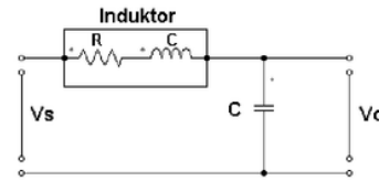
Gambar 2. Rangkaian filter pasif pelewat rendah LC
