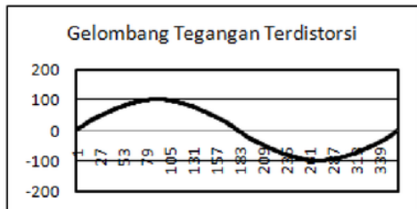
Gambar 11. Gelombang tegangan terdistorsi harmonik pada Lampu Hemat Energi setelah dipasang tapis LC.
