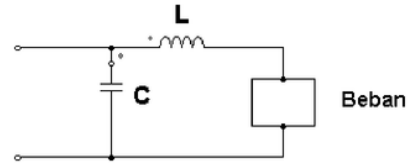
Gambar 8. Rangkaian Tapis Pasif LC yang digunakan pada Penelitian
