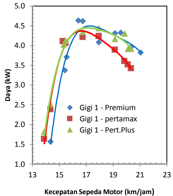
Gambar 4. Karakteristik daya terhadap kecepatan sepeda motor di gigi satu
