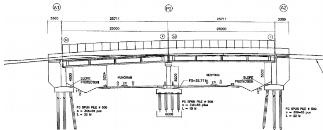
Gambar 2.1 Tipikal Struktur Jembatan
