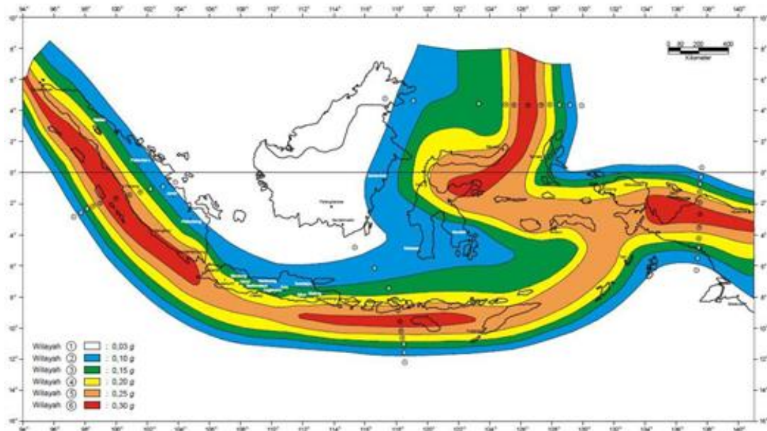
Gambar 2.7 Lokasi Pembagian Daerah Gempa
