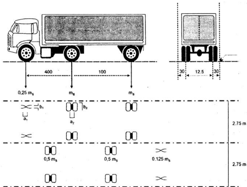
Gambar 2.6 Ketentuan beban “T” yang dikerjakan pada jembatan jalan raya
