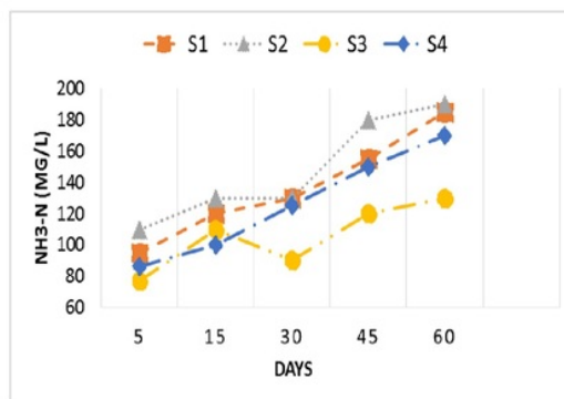
Fig. 6. \text{NH}_3\text{-N} value
