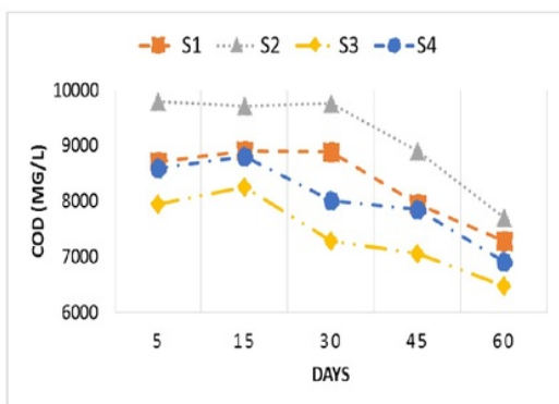
Fig. 5. COD value
