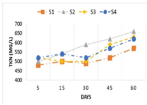
Fig. 7. TKN value.
