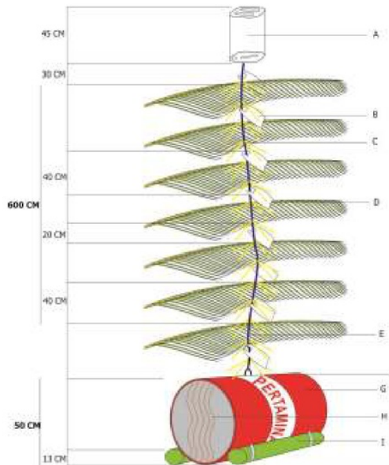
Gambar 1. Konstruksi rumpun yang digunakan dalam penelitian
