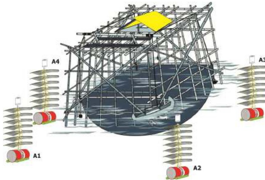
Gambar 2. Gambaran penempatan rumpon pada bagan
