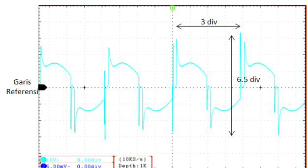
Gambar 16. Gelombang tegangan keluaran inverter half-bridge tanpa filter pasif beban dinamis
