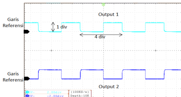
Gambar 8. Gelombang keluaran IC SG3524
