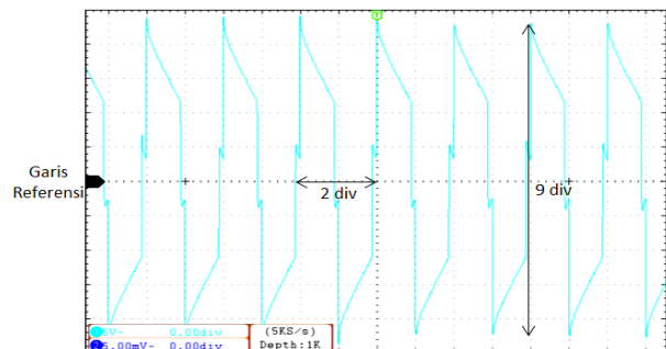
Gambar 10. Gelombang tegangan keluaran inverter half-bridge tanpa filter pasif beban resistif 289,5 \Omega
