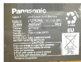
Gambar 3. Baterai 12V 7Ah
