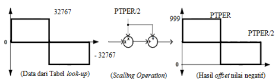
Gambar 9. Proses normalisasi sinyal referensi
