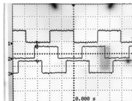
Gambar 13. Beda fase 120^\circ PWM1H, PWM2H dan PWM3H
