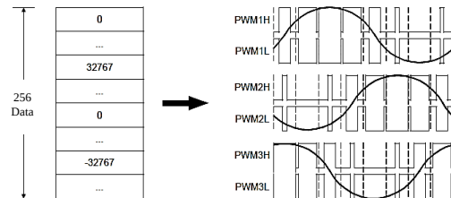
Gambar 8. Sinyal sinusoidal tiga fase dengan look-up table
