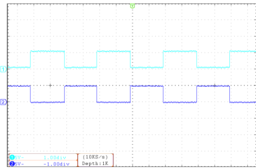
Gambar 11. Output PWM1L dan PWM1H
