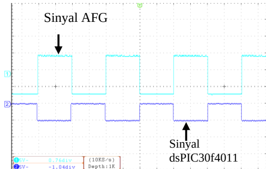
Gambar 14. PWM 50 Hz
