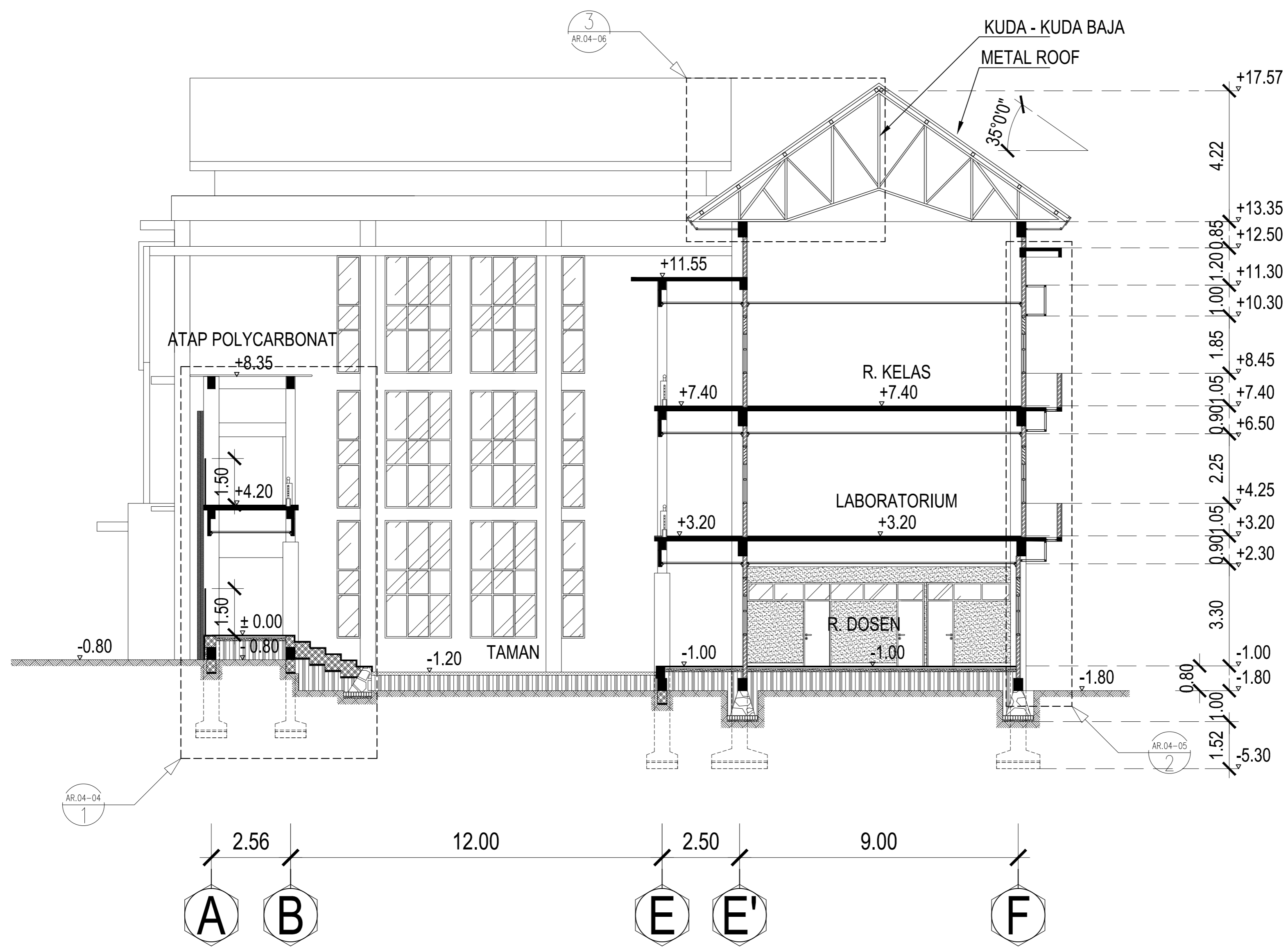
AR.04-01 POTONGAN A 1:150
