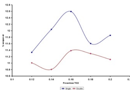
Gambar 4 Grafik hubungan pengaruh penambahan TiO 2 terhadap persentase serapan air
