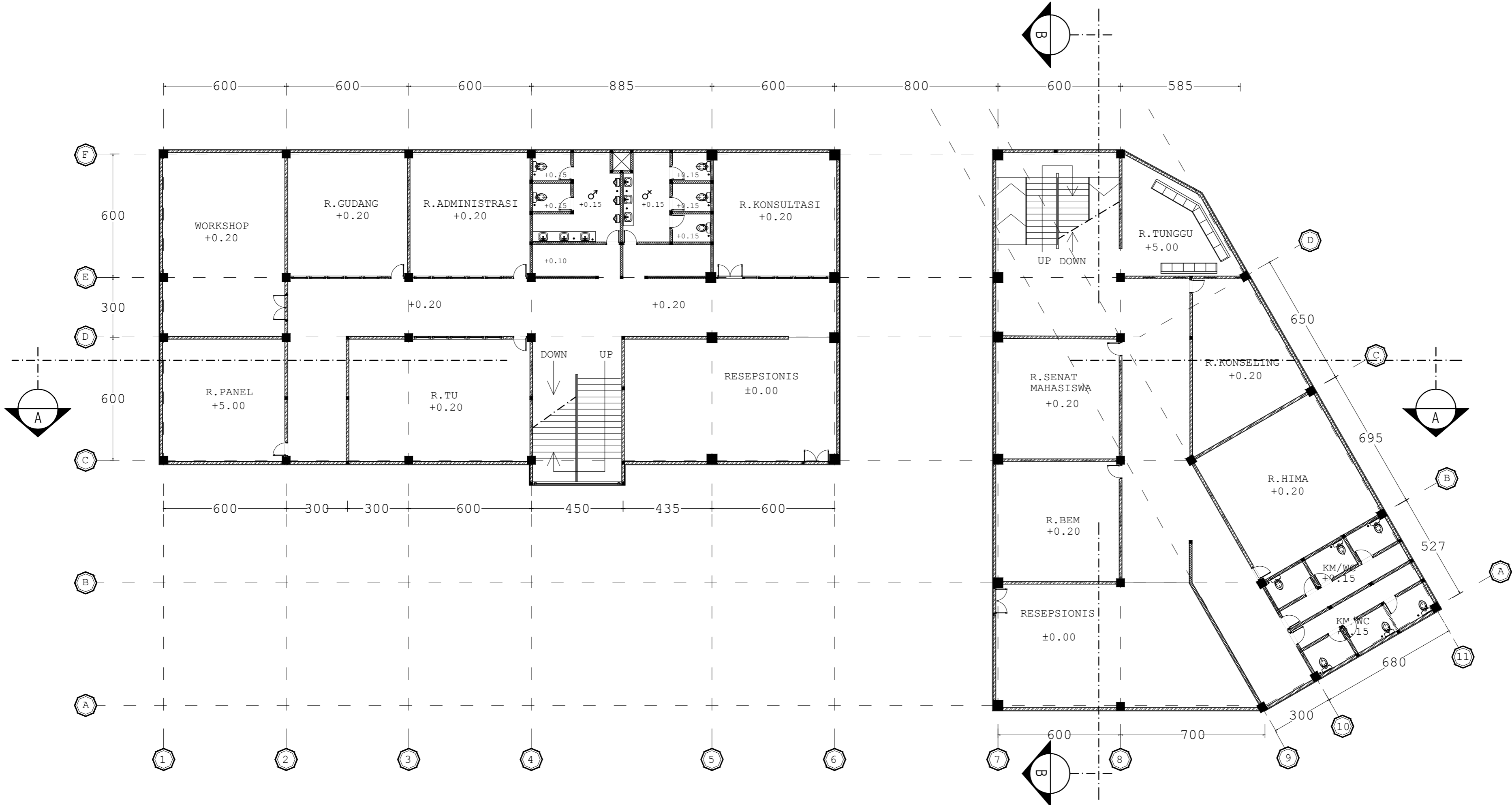
02 DENAH LT. 1 REF SKALA 1:150
