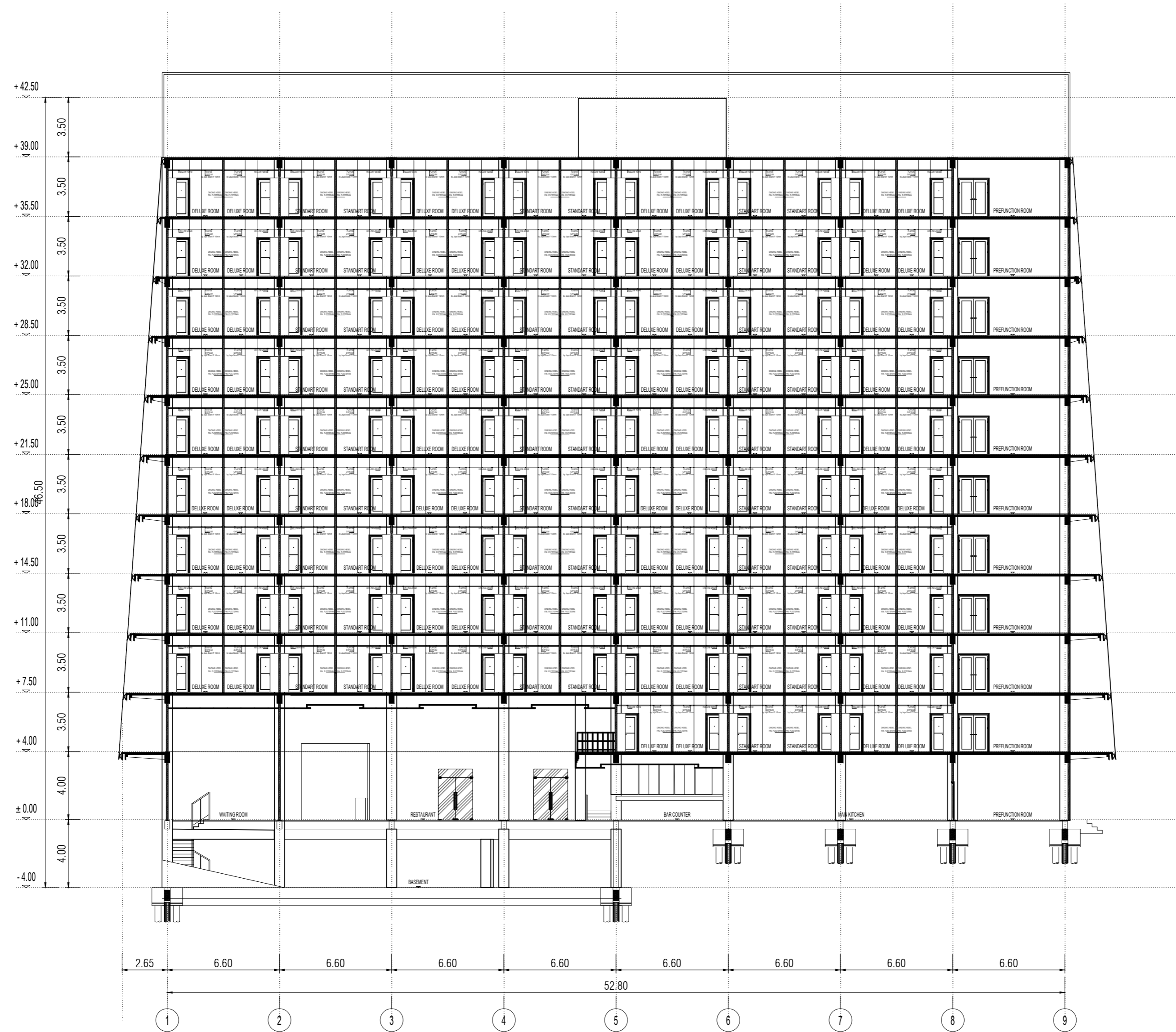
1 POTONGAN A-A AR 11 1:200
