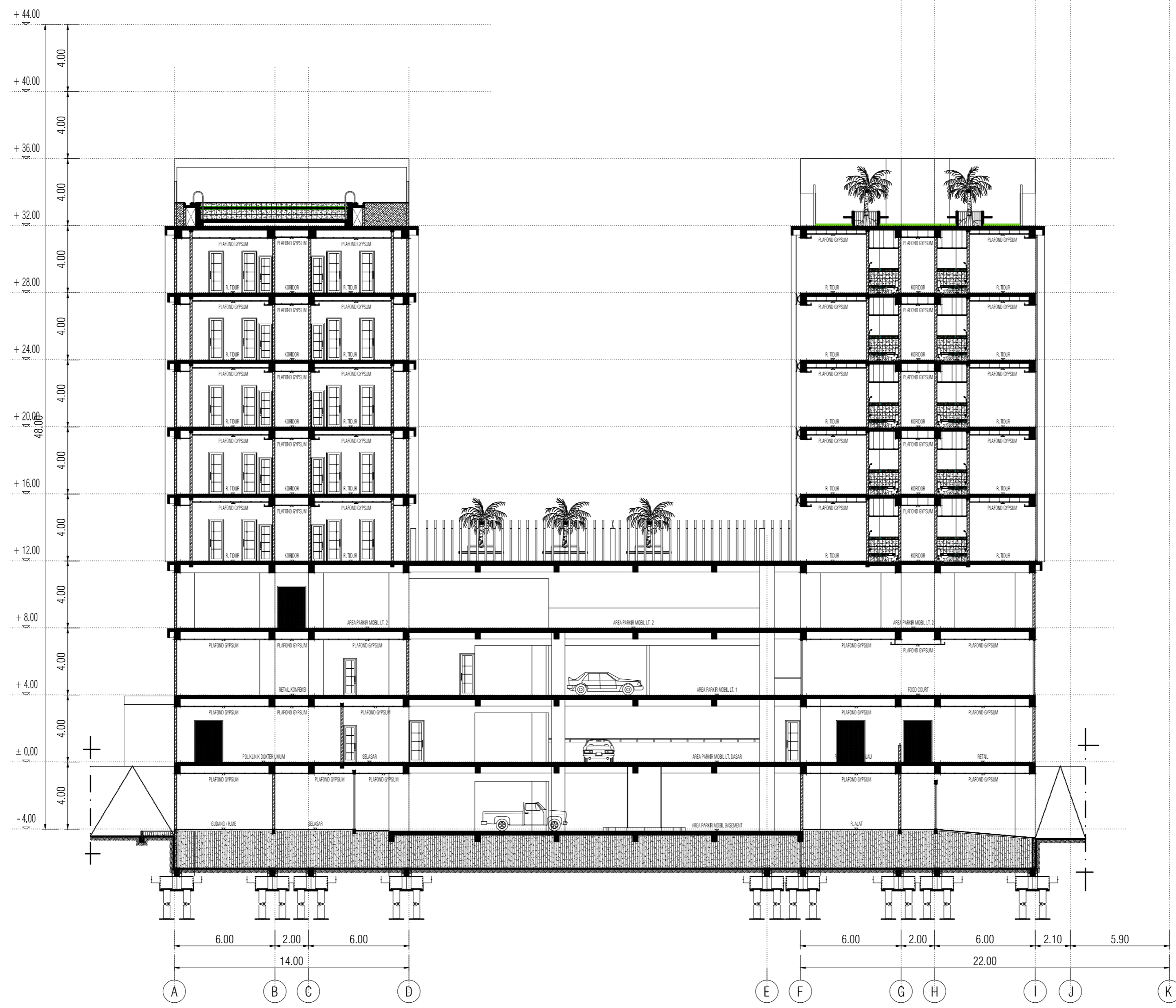
1 POTONGAN B-B 29 1:200
