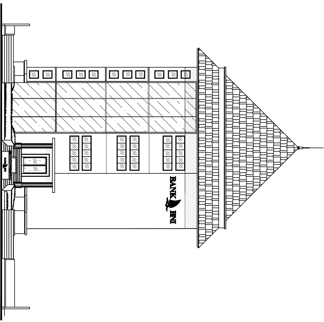
TAMPAK DEPAN skala 1:100
