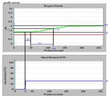
Gambar 10 Tanggapan kelauran sistem pengendalian pH berdasarkan uji bumpstest .
