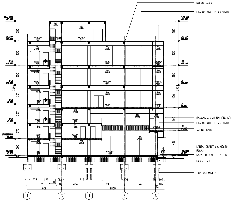
01 POTONGAN A-A AR.04 SKALA 1:150
