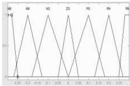
Gambar 7 Fungsi keanggotaan Error
