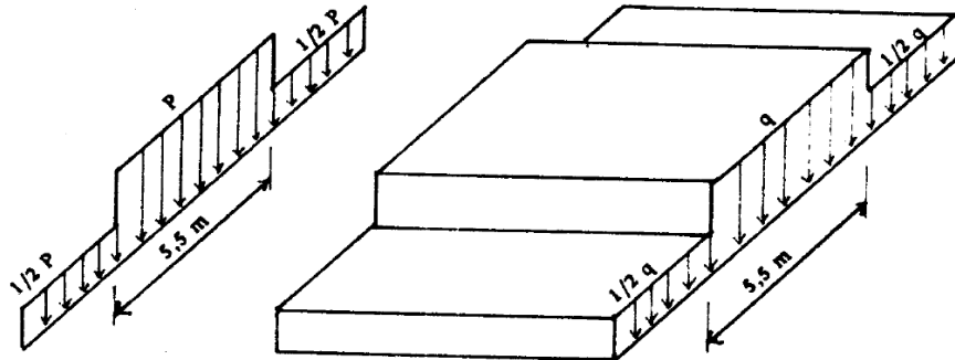
Gambar 2.3 Ketentuan Penggunaan Beban “D”
