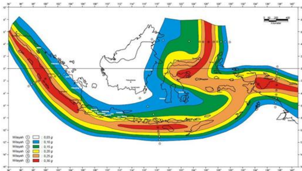
Gambar 2.4 Lokasi Pembagian Daerah Gempa
