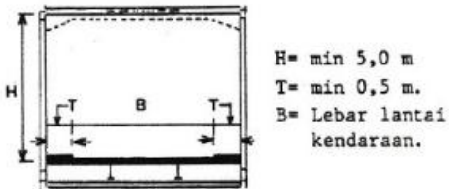
Gambar 2.7 Lebar maksimum jembatan
