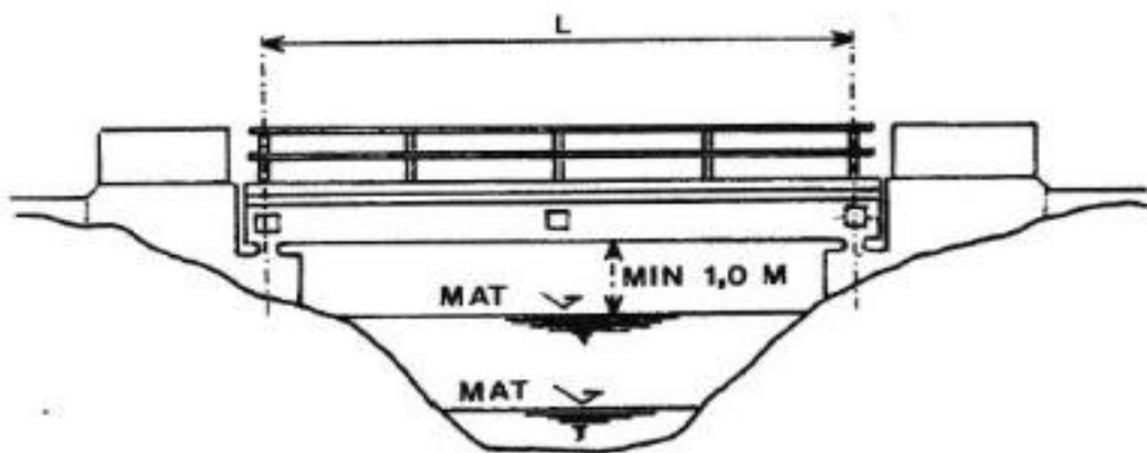
Gambar 2.8 Tinggi bebas maksimum terhadap banjir 50 tahunan
