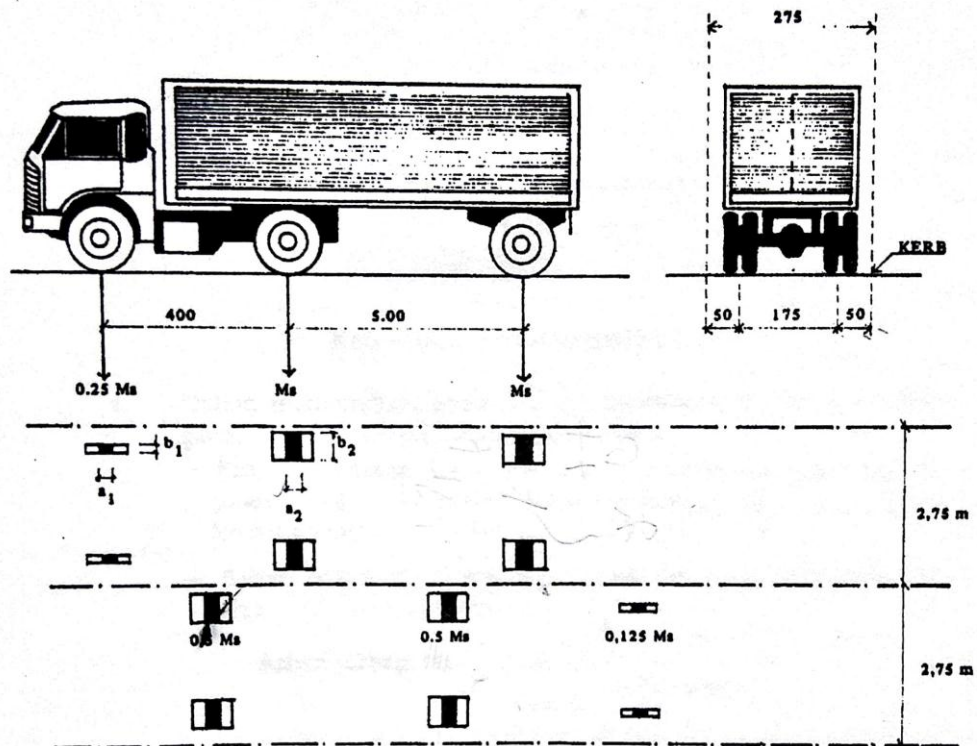
Gambar 2.1 Jumlah Jalur Lalu Lintas
