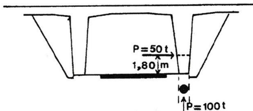
Gambar 2.5 Gaya Tumbuk Pada Jembatan Layang
