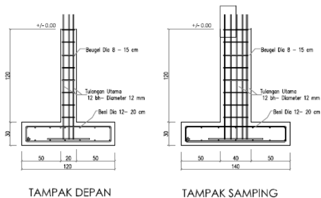
Gambar 2. 2 Pondasi Plat
