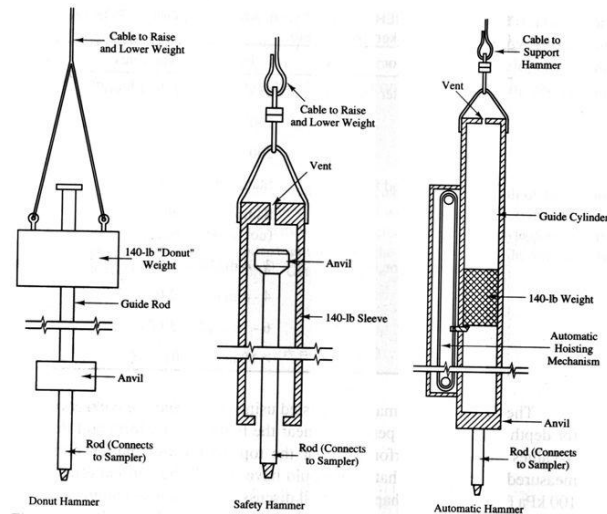
Gambar 2. 12 Tipe Pemukul SPT
