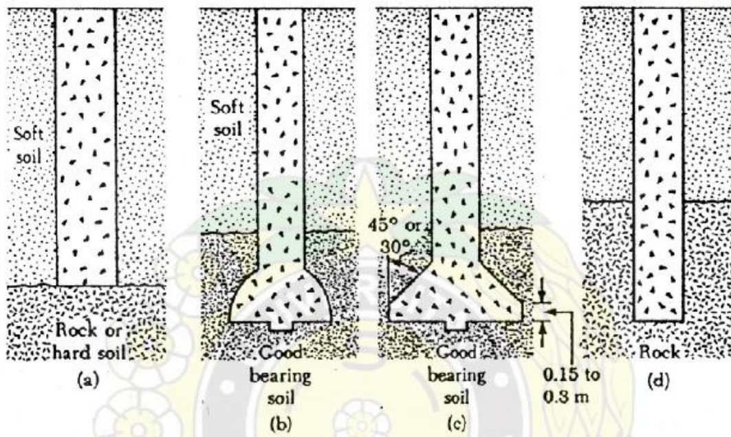
Gambar 2. 9 Jenis-Jenis Bore Pile
