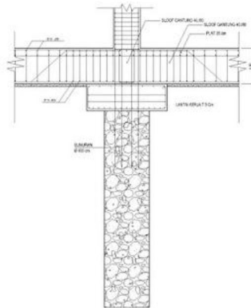
Gambar 2. 4 Pondasi Sumuran
