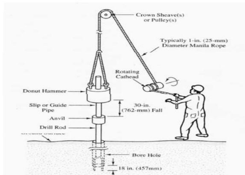
Gambar 2. 11 Uji SPT secara manual
