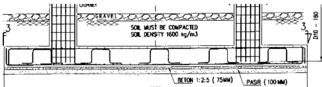
Gambar 2. 5 Pondasi Rakit
