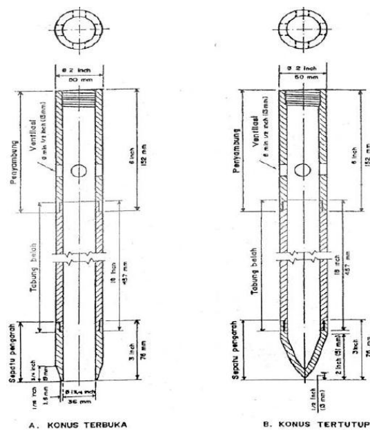
Gambar 2. 10 Tabung Belah
