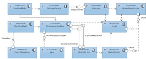
Gambar 16. Component diagram dari sistem yang akan dibangun
