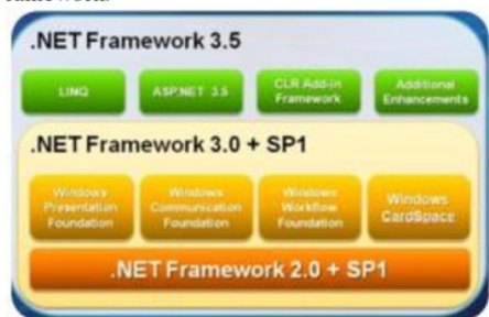
Gambar 1. WPF di dalam .Net Framework 3.5
