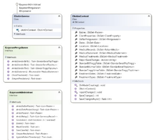
Gambar 5. Class diagram dari lapisan Data Access Layer
