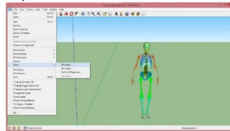
Gambar 9 Ekspor Objek
