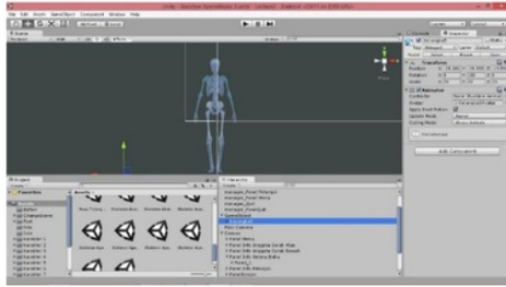
Gambar 11 Inspektor Objek
