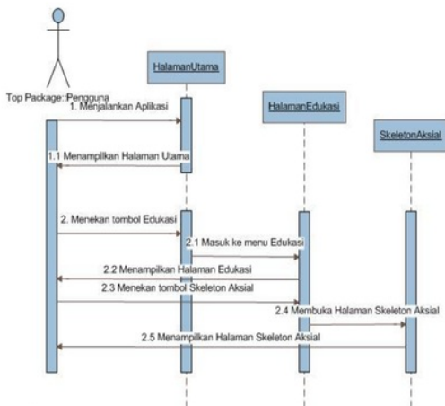
Gambar 6 Diagram Sequence untuk use case menekan Tombol Skeleton Aksial
