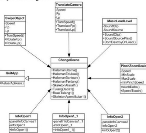
Gambar 8 Diagram Kelas
