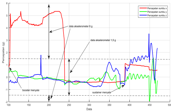
Gambar 6. Percepatan gerak roket dengan menggunakan algoritme PDS.
