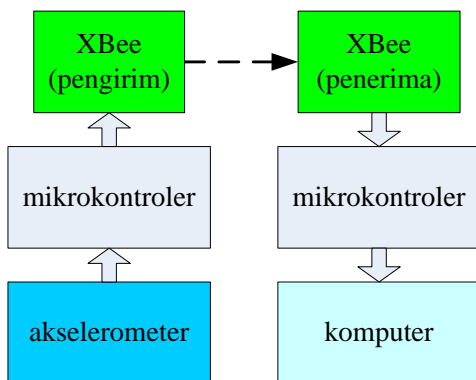
Gambar 2. Diagram blok perancangan perangkat keras sensor IMU.
