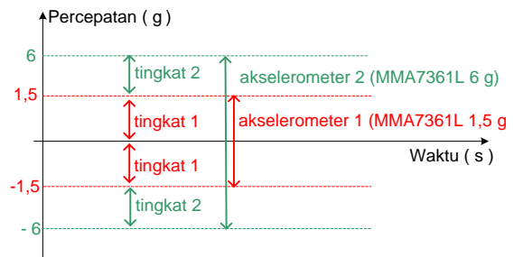
Gambar 5. Tingkat sensor percepatan.
