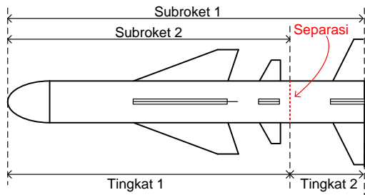
Gambar 1. Konfigurasi roket kendali.
