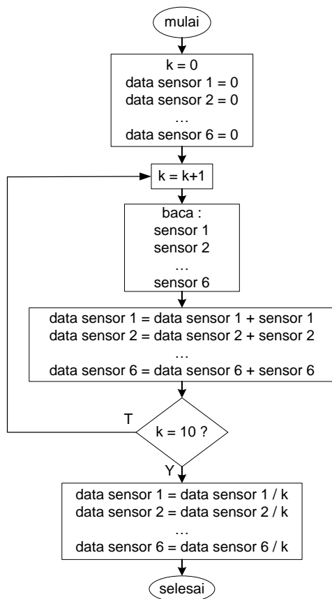
Gambar 4. Diagram alir filter moving average pada data sensor.
