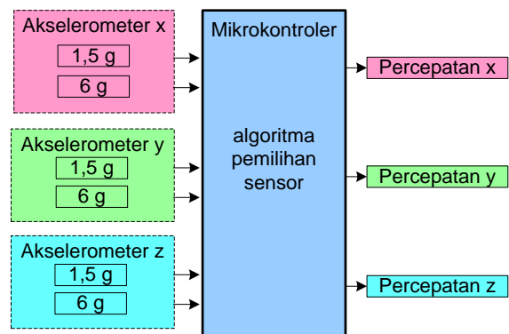
Gambar 3. Hubungan antara sensor dan mikrokontroler.
