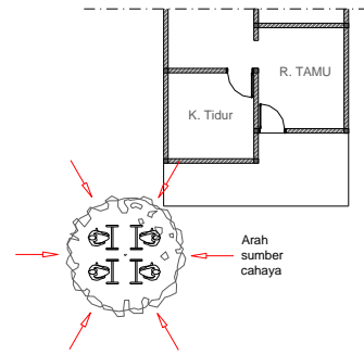
Gambar 14. Sumber cahaya pada halaman Sumber : Analisa Penelitian, 2017
