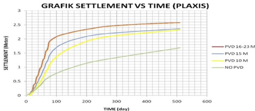
Gambar 13. Grafik Displacement Vs Time berbagai kedalaman PVD.
