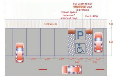
Gambar 22. Parkir Difabel menurut FIBA
