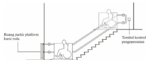
Gambar 16. Lif Tangga menurut Permen PUPR RI
