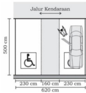
Gambar 23. Parkir Difabel menurut Permen PUPR
