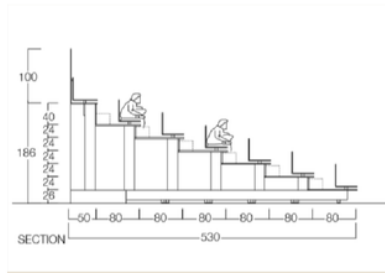
Gambar 26. Tribun menurut FIBA
