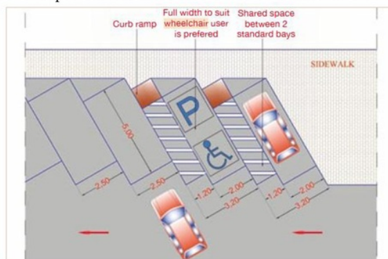
Gambar 21. Parkir Difabel menurut FIBA
