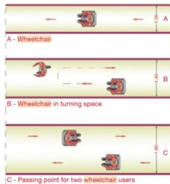
Gambar 7. Lebar Koridor menurut FIBA
