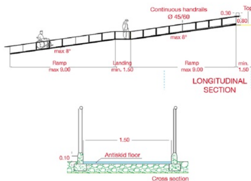
Gambar 8. Ram menurut FIBA
