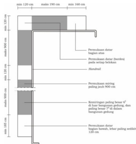
Gambar 9. Ram menurut Permen PUPR RI
