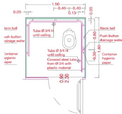
Gambar 19. Denah Toilet Difabel menurut FIBA
