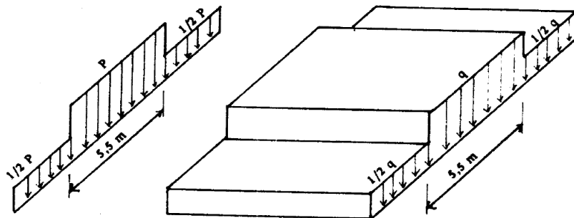
Gambar 2.3 Ketentuan Penggunaan Beban “D”
