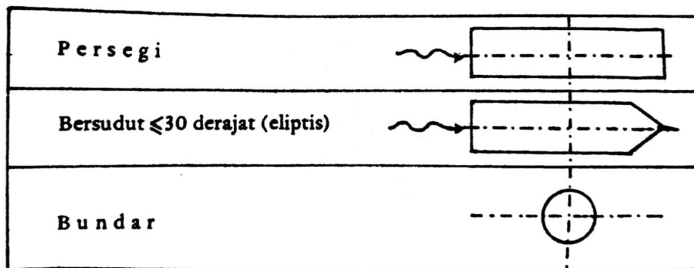
Gambar 2.5 Bentuk/Denah Pilar
