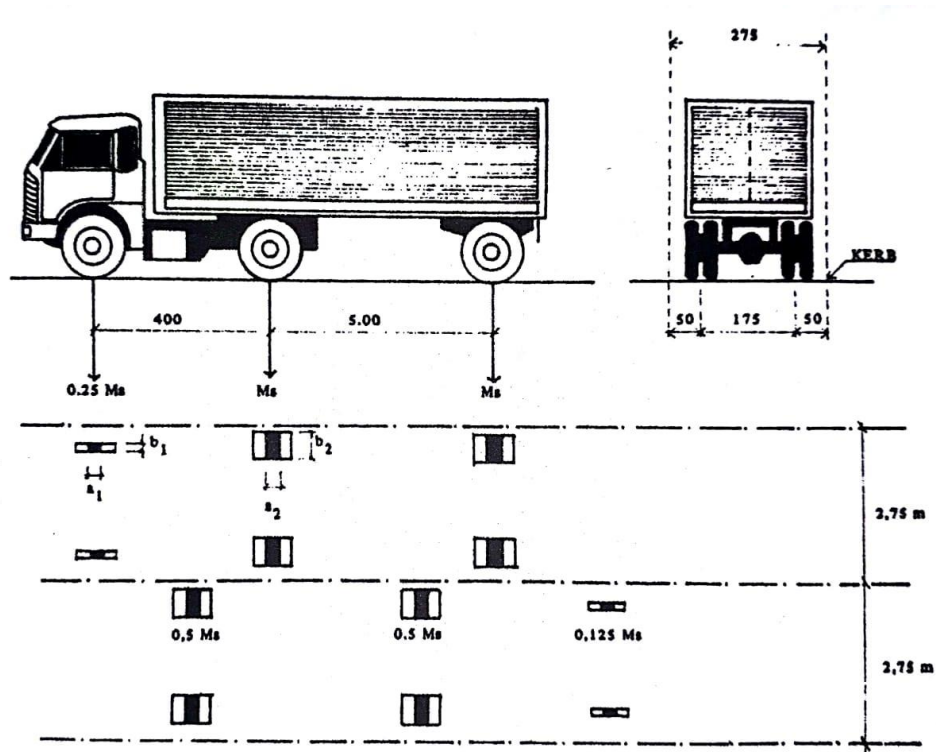
Gambar 2.1 Beban T
