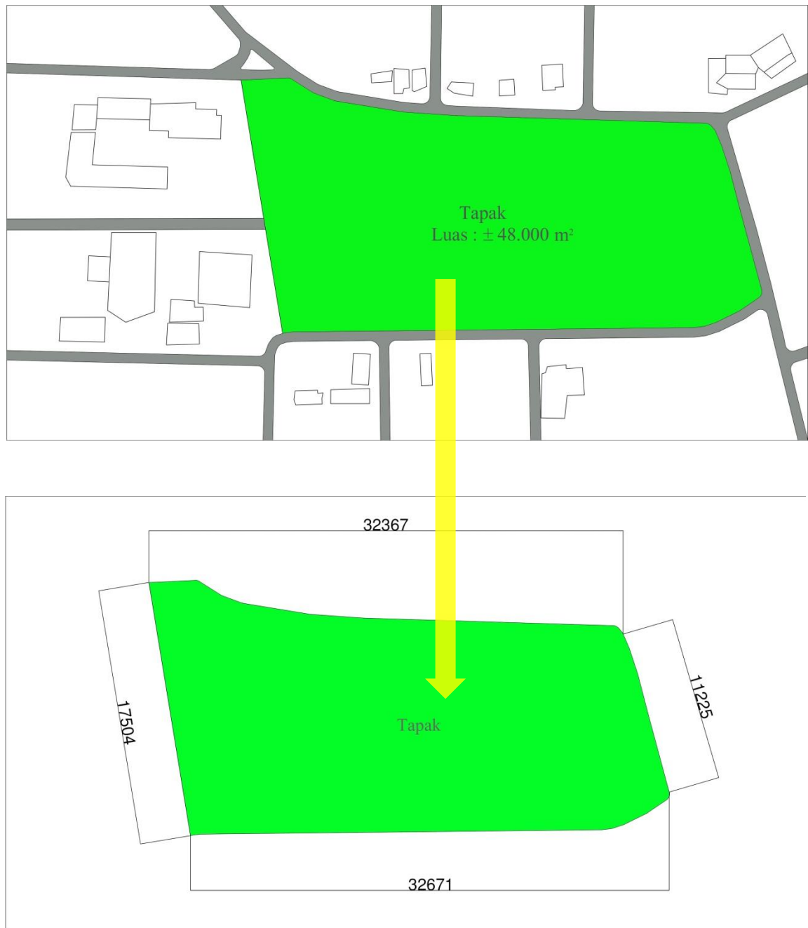
Gambar 6.2 Situasi dan ukuran tapak area UNDIP Pleburan Sumber : Gambar Pribadi
