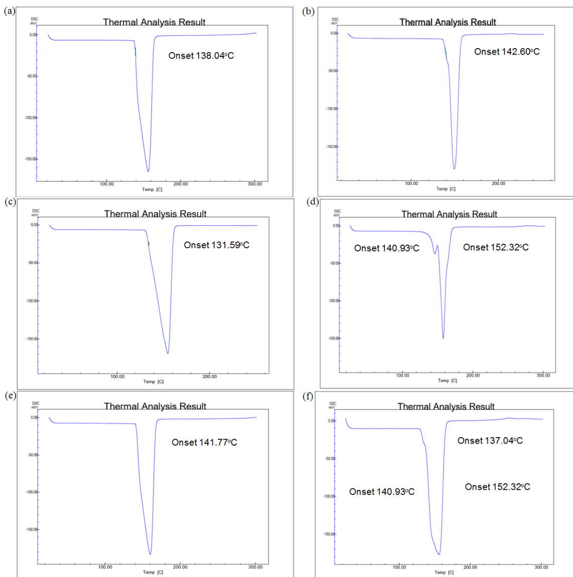
Figure 1. DSC Thermogram (a) alginate (b) κ-carrageenan (c) maltodextrin (d) FM (e) FMA (f) FMC
