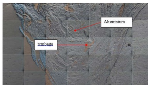
Gambar 8. Foto Makro FSW 1000 rpm
