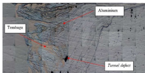
Gambar 7. Foto Makro FSW 800 rpm
