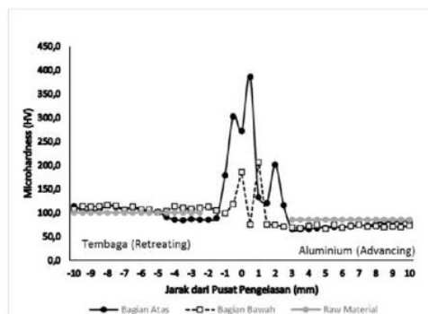
Gambar 5. Distribusi kekerasan mikro pada pengelasan dengan kecepatan putaran pahat 800 rpm
