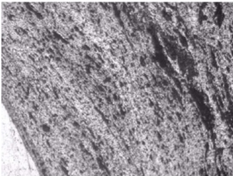
Gambar 10. Foto Mikro TMAZ 1000 rpm
