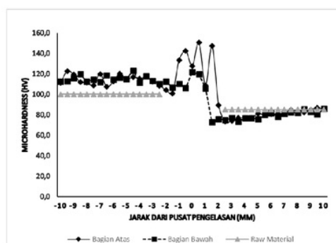
Gambar 6. Distribusi kekerasan mikro pada pengelasan dengan kecepatan putaran pahat 1000 rpm
