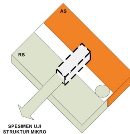
Gambar 3. Pengambilan spesimen uji kekerasan mikro dan struktur mikro
