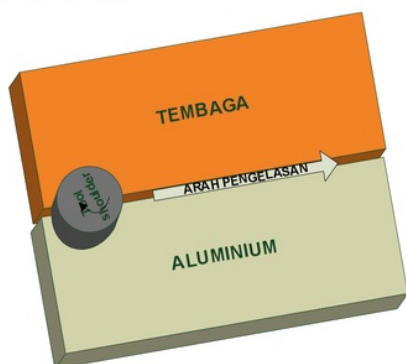
Gambar 1. Skema pengelasan FSW logam aluminium dan tembaga
